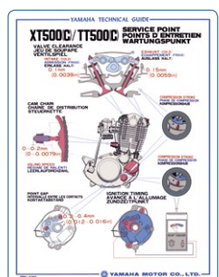
Wartungsplan Bestellnr. 80156
